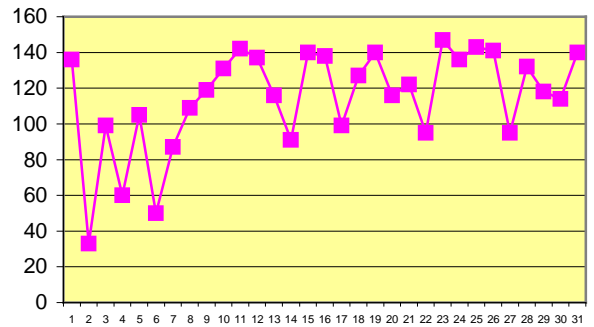
production journalière du mois de Juillet 2009 (kWh)
