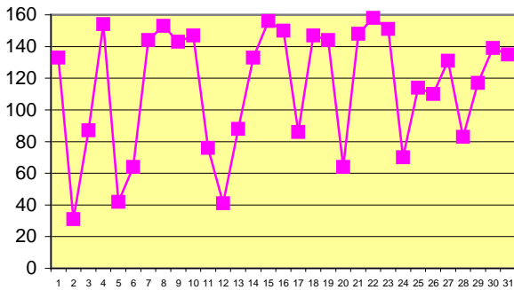
production journalière du mois de Juillet 2008 (kWh)
